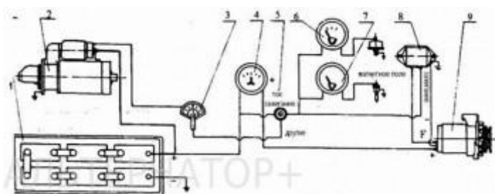
Рис. 8. Электрическая схема
