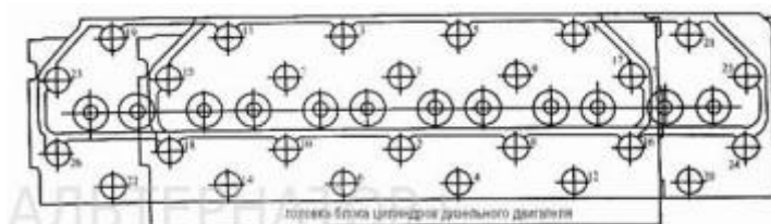
Рис. 1. Последовательность затяжки болтов головки блока цилиндров
