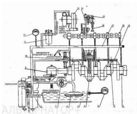
Рис. 6 Схема смазочной системы
